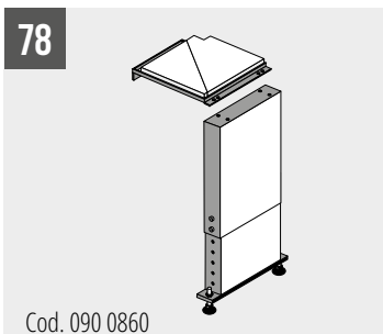
SHARK 382-1 SXI evo Adattatore lato scarico
