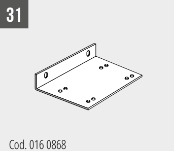
COBRA 352 MA Adattatore lato scarico
